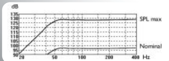
Réponse en fréquence / Frequency response
